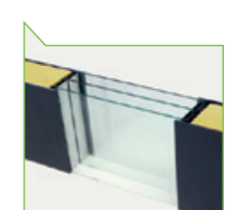
Standard 3 Scheiben Wärmeschutzglas (U Wert=0,5 - 0,6 W/m²K)
