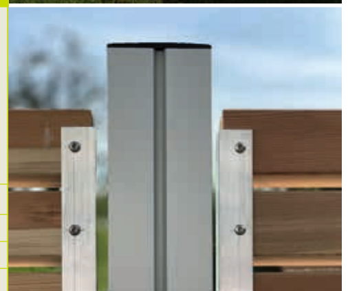
Sichtschutz ASL 6060 in Kombination mit APIARY R Seite 90
