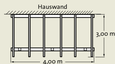
Planungsbeispiel einer Pergola ohne Pergolaverbinder
